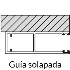
Instalación guía
